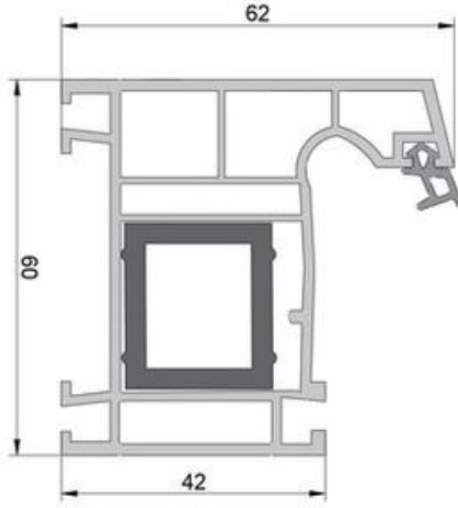
ES 010 L Kasa Profili L Frame Profile
