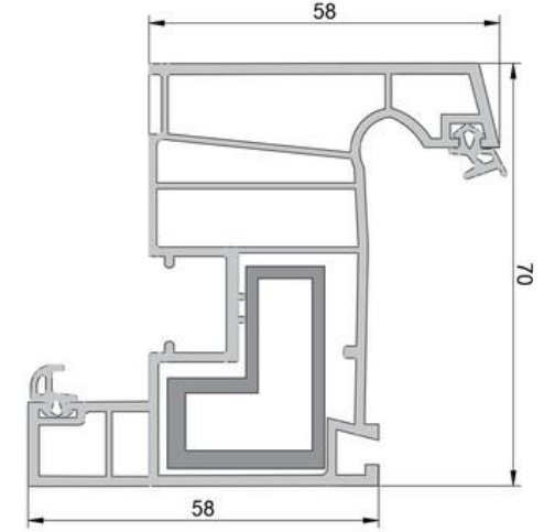
OKS 030 Pencere Kanat Profili Window Sash Profile
