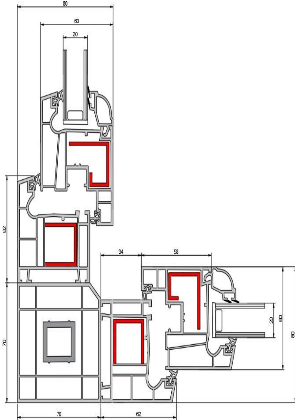
90 Derece Birleşim Detayı 90 Degree Connection Detail
