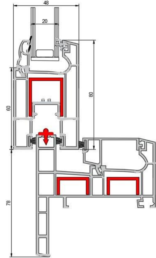
Sabit Sürme-Kanat Kapama Profili Birleşim Detayı Sliding Fixed_-Sash Closing Profile Connection Detail
