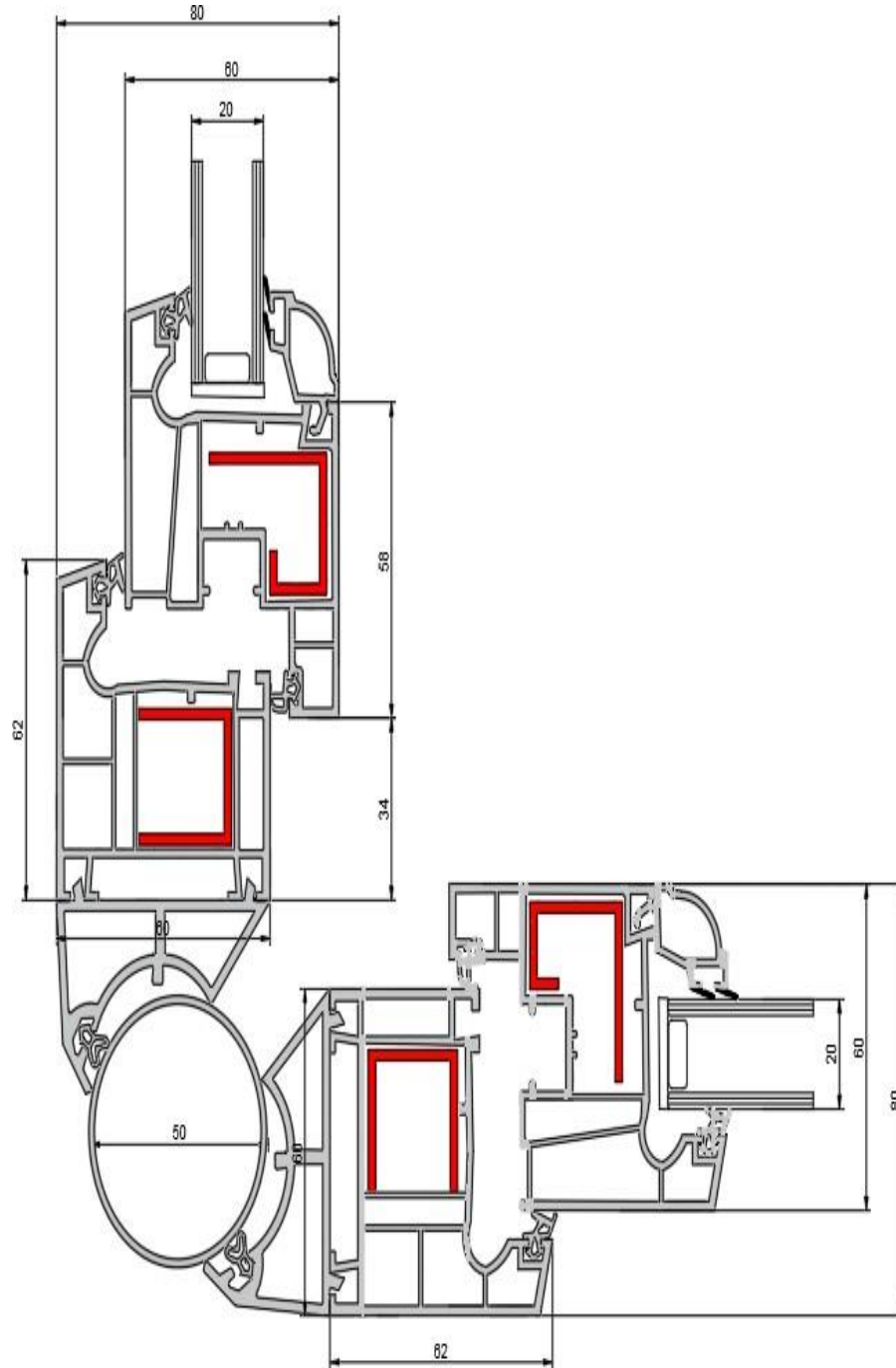
Köşeli Birleşim Detayı Angular Connection Detail
