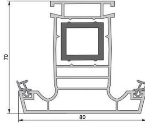
OKS 020 Orta Kayıt Profil Mullion Profile
