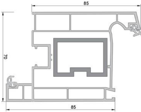
OKS 040 Kapı Kanat Profili Door Sash Profile
