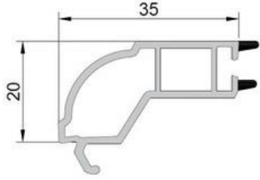
OP 01 Tek Cam Çıtası Single Glazing Bead
