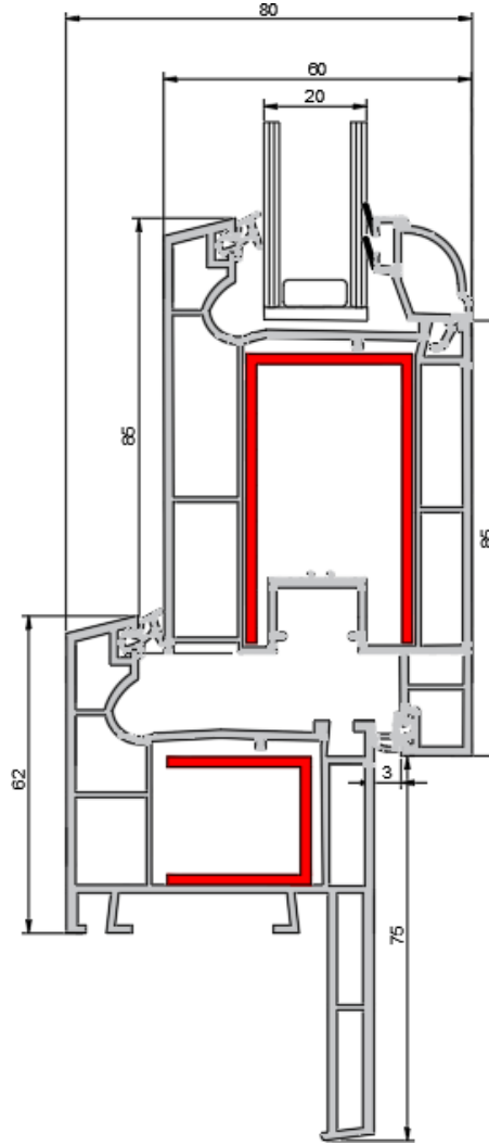
Kasa - Pencere Kanat Birleşim Detayı Flame - Window Sash Connection Detail
