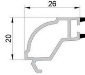
OP 08 Çift Cam Çıtası Double Glazing Bead
