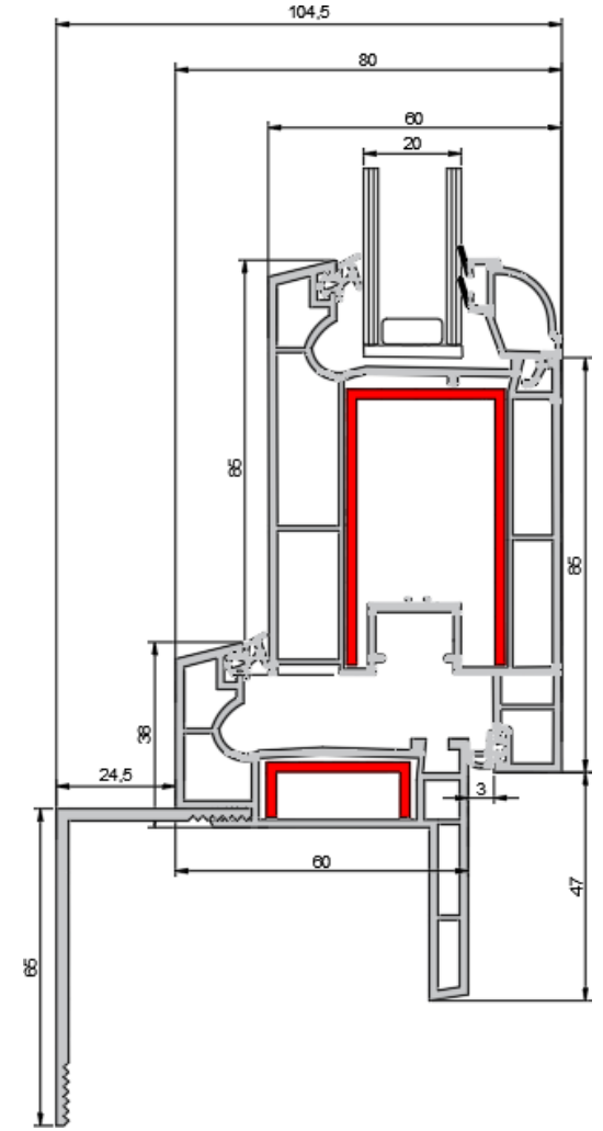
Pervazlı Kasa-Kapı Kanat Birleşim Detayı Renovation Frame-Door Sash Connection Detail
