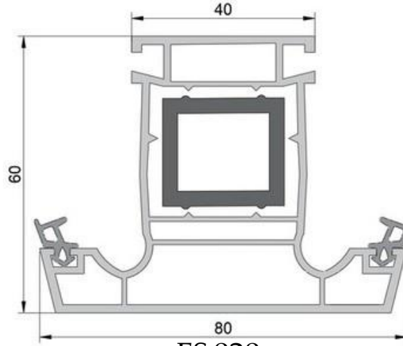
ES 020 Orta Kayıt Profili Mullion Profile
