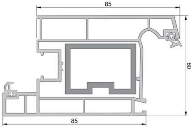
ES 040 Kapı Kanat Profili Door Sash Profile
