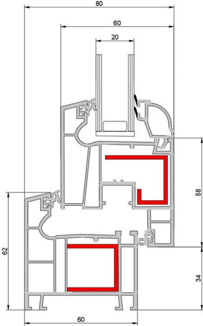
Kasa - Pencere Kanat Birleşim Detayı Flame - Window Sash Connection Detail
