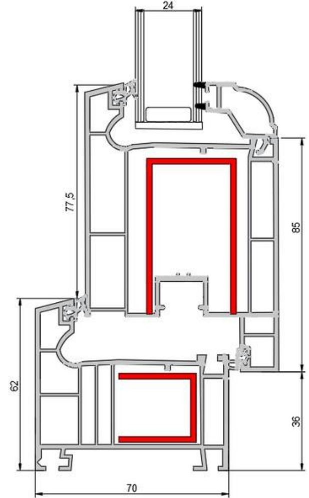
Kasa-Kapı Kanat Birleşim Detayı
