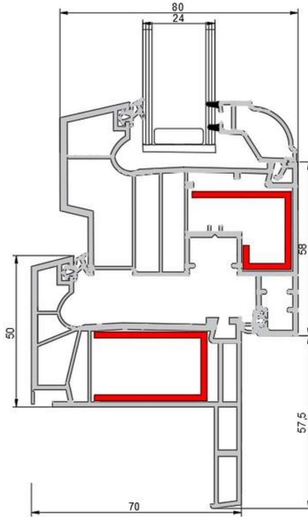
Pervazlı Kasa-Damlalık Kanat Birleşim Detayı
