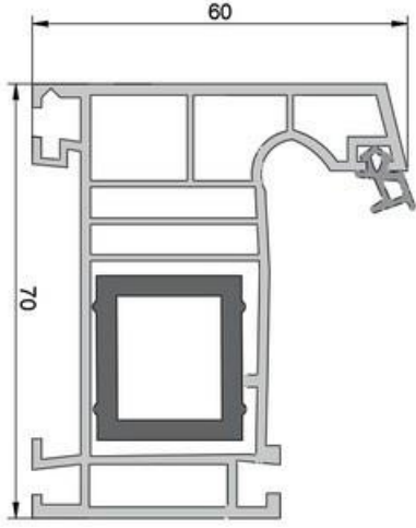
OKS 010 Kasa Profili Frame Profile
