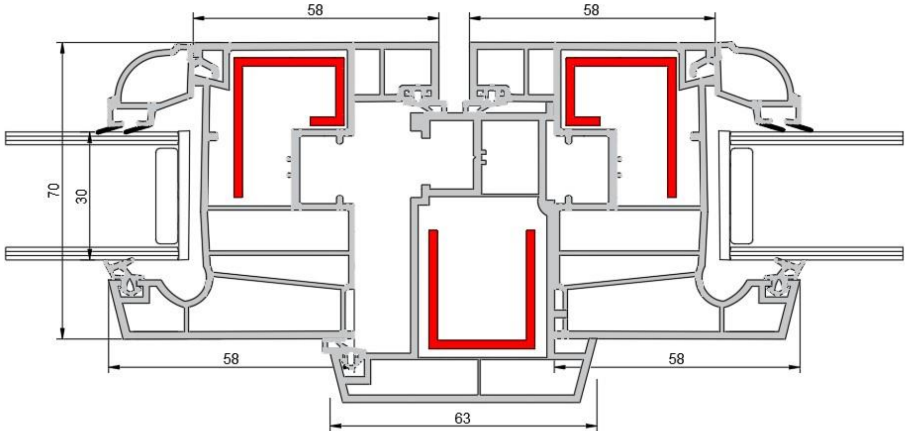
Hareketli Orta Kayıt-Kanat Birleşim Detay1 Sliding Mullion Profile-Sash Connection Detail
