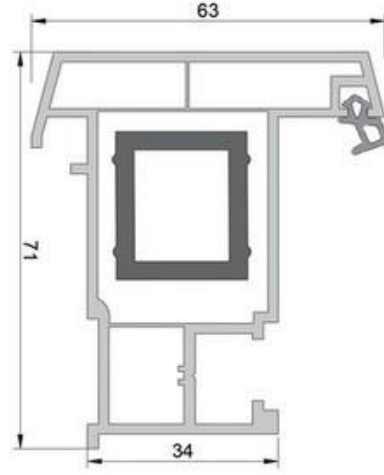
OKS 080 Hareketli Orta Kayıt Sliding Mullion Profile
