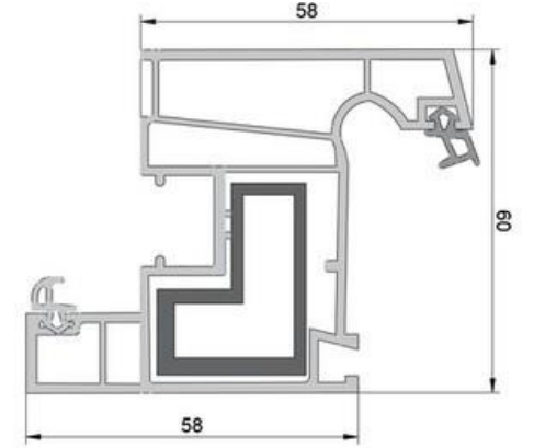
ES 030 Pencere Kanat Profili Window Sash Profile
