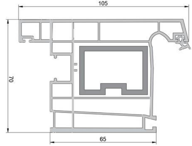
OKS 090 Dışa Açılır Kapı Kanat Prof. Outward Door Sash Prof.
