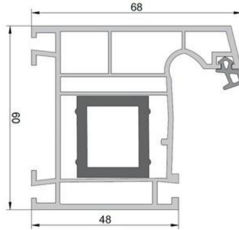
ES 050 Süper Kasa Profili Super Frame Profile
