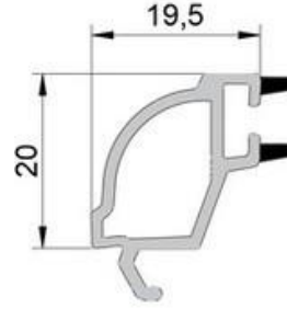
OP 02 Çift Cam Çıtası Double Glazing Bead
