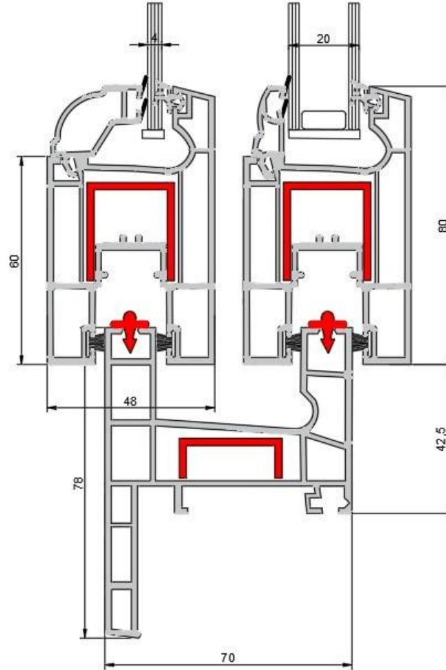
Sliding Frame-Sash Birleşim Detayı Sliding Frame-Sash Connection Detail
