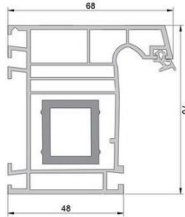
OKS 050 Süper Kasa Profili Super Frame Profile
